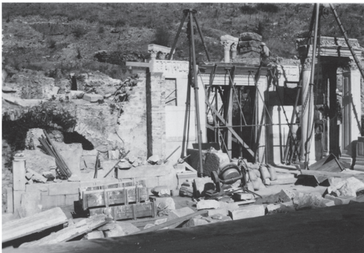
2 Wiederaufbau des ›Hadrianstempels‹, Schalung im oberen Bereich der Cella-Südwand
