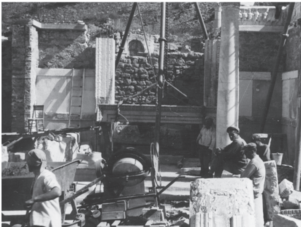
2 Versetzen des Türsturzes am Tempel
