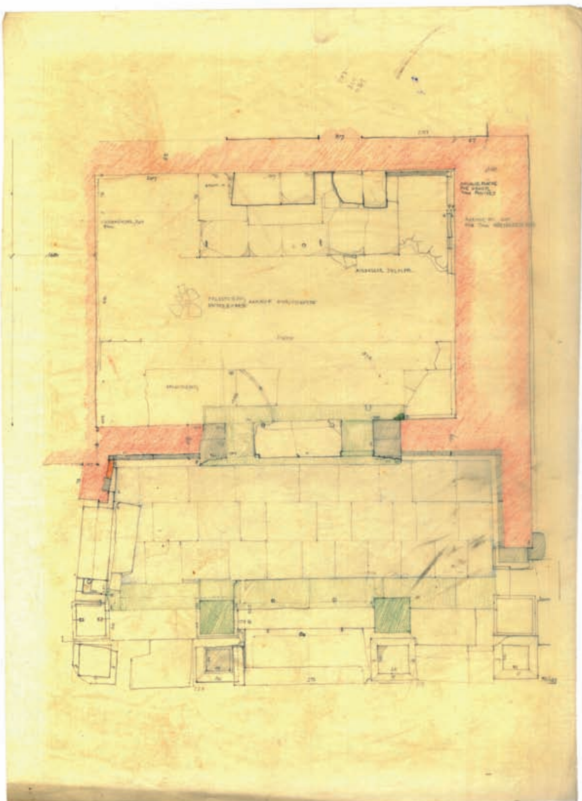
Zeichnerische Aufnahme des Grundrisses von K. H. Göschl, 1956 (?)
