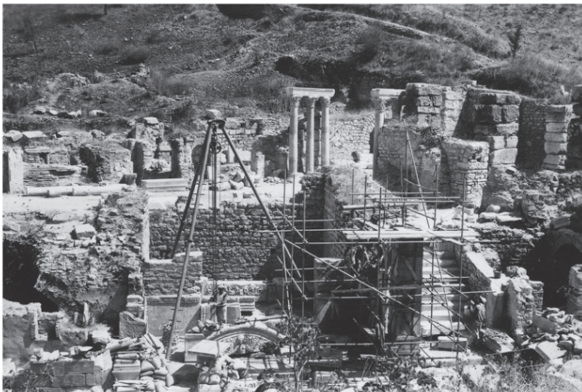
1 Wiederaufbau des ›Hadrianstempels‹, Schalung des östlichen Pfeilers vor Ort
